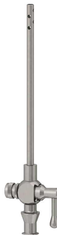
VED-329901-32 Spülkanüle mit Hahn, Trokar, Obturator, Ø 3,2 mm, Luer-Lock Anschluss, Arbeitslänge 70 mm
